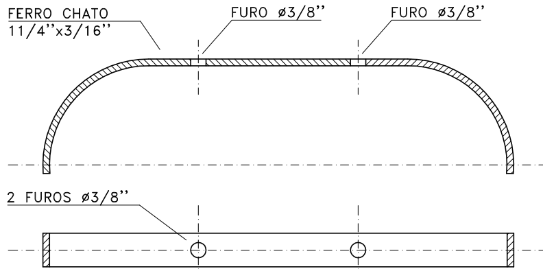
SUPOORTE INTERNO PARA DUTO GIROVAL LADO MAIOR ATÉ \phi 557\text{mm}
