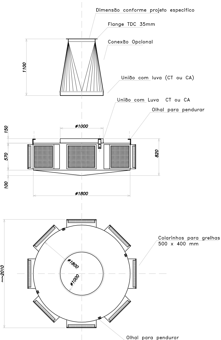
CAIXA DIFUSORA DE AR PARA 08 GRELHAS PADRÃO REFRIN
